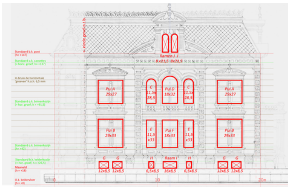
Oorspronkelijke tekening uit 1895 van de verbouwing tot villa, met daarop ingetekend de diverse merken van de 3D prints [Afbeelding van de auteur]
